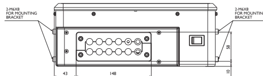
喷码机支架
