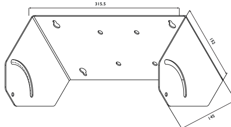
喷码机支架
