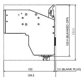
紧凑型打印头 - 上插口
