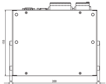
OPT打印头 - 上插口
