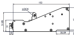
EXT打印头 - 上插口
