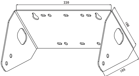
마킹기 브래킷
