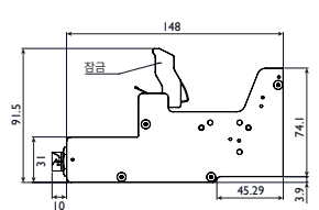
OPT 프린트 헤드 - 상단 커넥터
