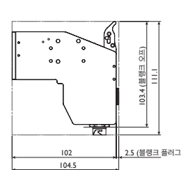
소형 프린트 헤드 - 상단 커넥터
